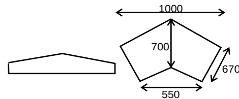
Riska PIER CAP
